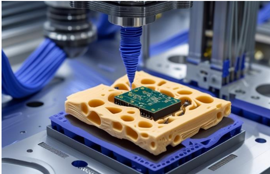
Figura 4. Imagem processo de impressão DIW: extrusão de tinta com grafeno criando um circuito eletrônico (autoral)
